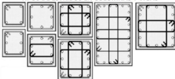
TIPOS DE ESTRIBOS EN COLUMNAS Y VIGAS
